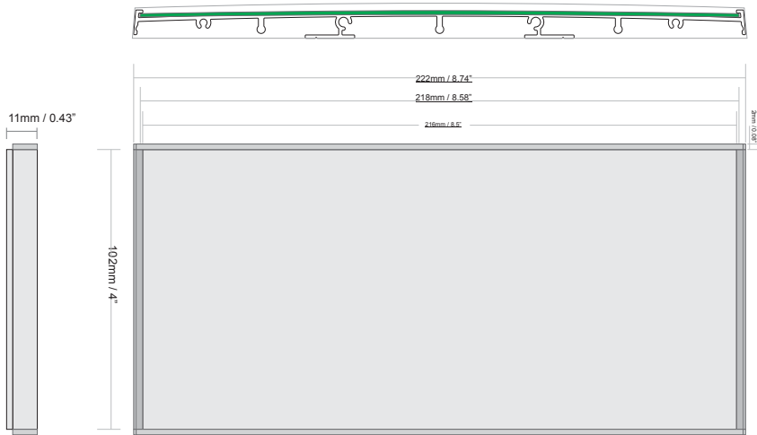
1. Room ID 4"x8.74" Mir 2409
